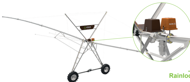
Опора с гидравлическим приводом Опора з гідравлічним приводом
