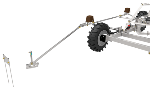
Направляющий башмак Напряний башмак
